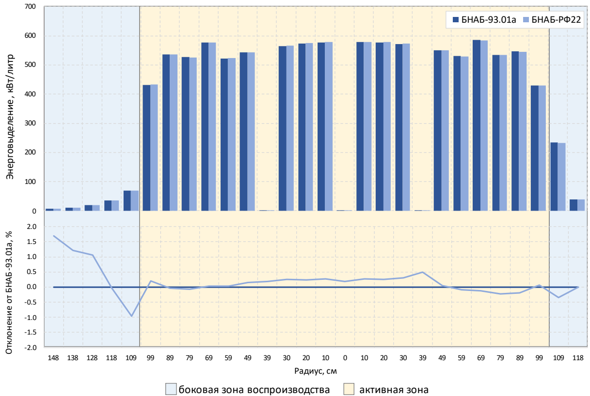
Рисунок 4.10 – Результаты расчета удельного энерговыделения по а.з. реактора БН-600 по системам констант БНАБ-93.01а и БНАБ-РФ22
