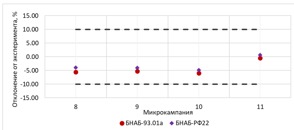
Рисунок 4.7 – Средние значения расчетно-экспериментальных отклонений эффективности стержней ПАЗ
