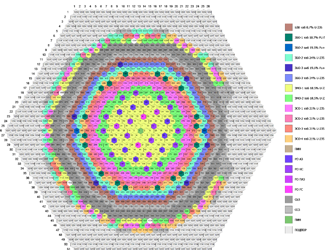
Рисунок 2.11 – Картограмма реактора БН-800 (8 микрокампания)
