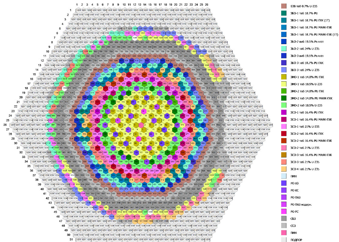
Рисунок 2.12 – Картограмма реактора БН-800 (9 микрокампания)
