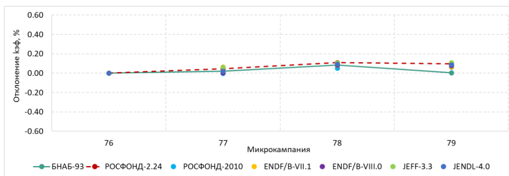
Рисунок 3.11 – Изменение значения k_{эф} по отношению к 76 микрокампании реактора БН-600
