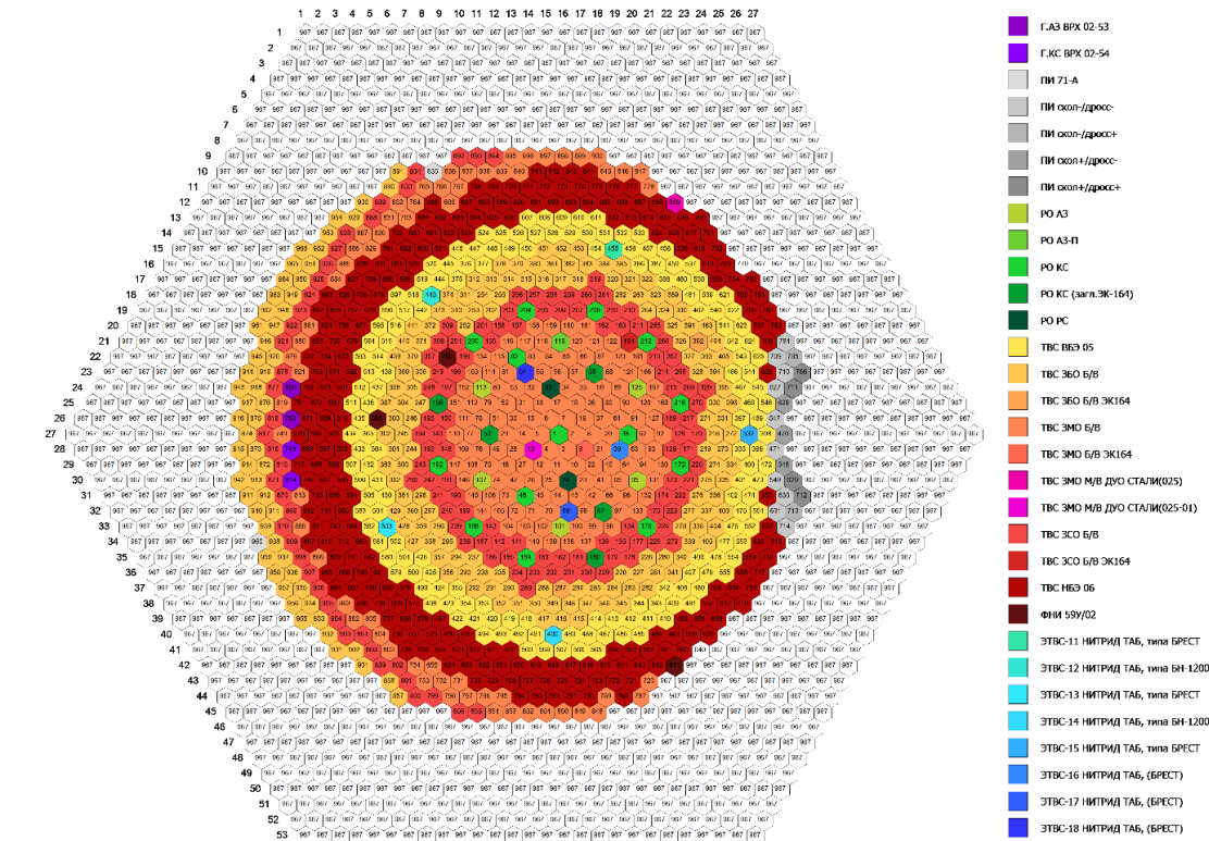
Рисунок 2.7 – Картограмма реактора БН-600 (76 микрокампания)
