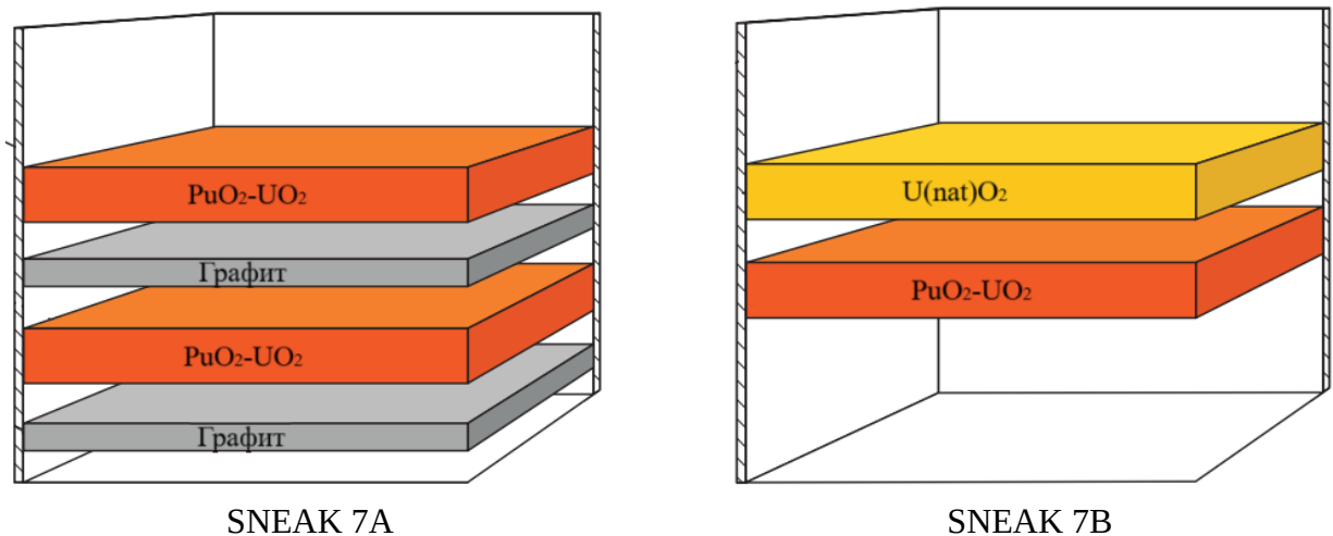
Рисунок 2.1 – Конфигурация сборок SNEAK 7A и 7B
