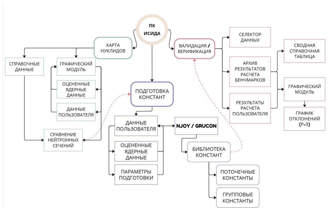
Рисунок 1.2 – Общая схема архитектуры ИСИДА
