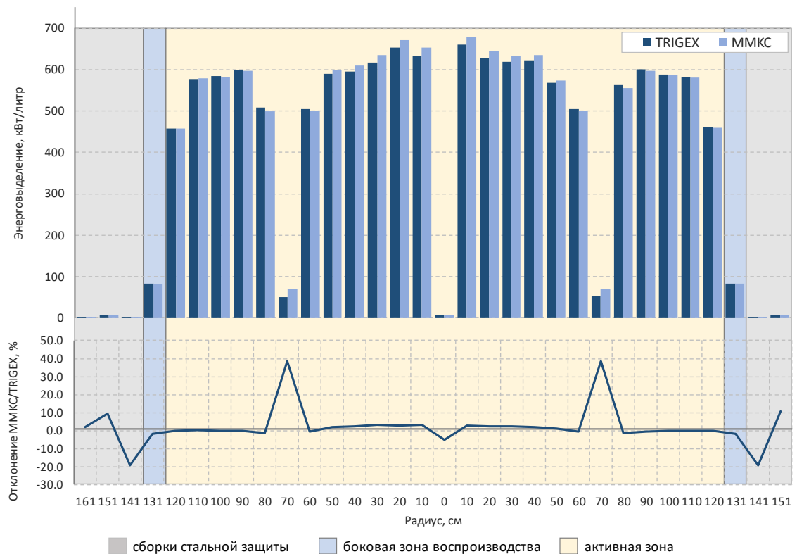
Рисунок 4.13 – Результаты методической поправки для удельного энерговыделения по радиусу активной зоны, 11 микрокампания РУ БН-800
