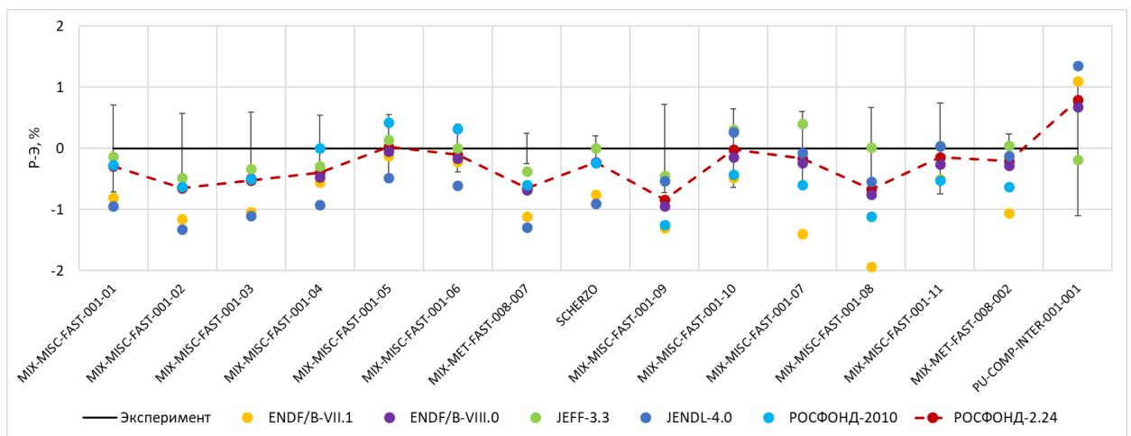
Рисунок 3.6 – Расчетно-экспериментальное отклонение для экспериментов с k_{\infty} близким к единице
