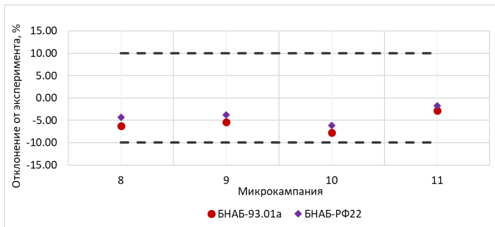
Рисунок 4.6 – Средние значения расчетно-экспериментальных отклонений эффективности стержней КС
