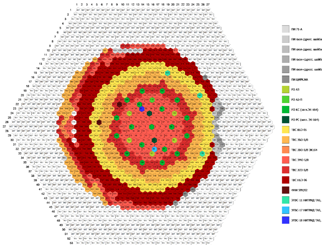
Рисунок 2.9 – Карттограмма реактора БН-600 (78 микроампания)
