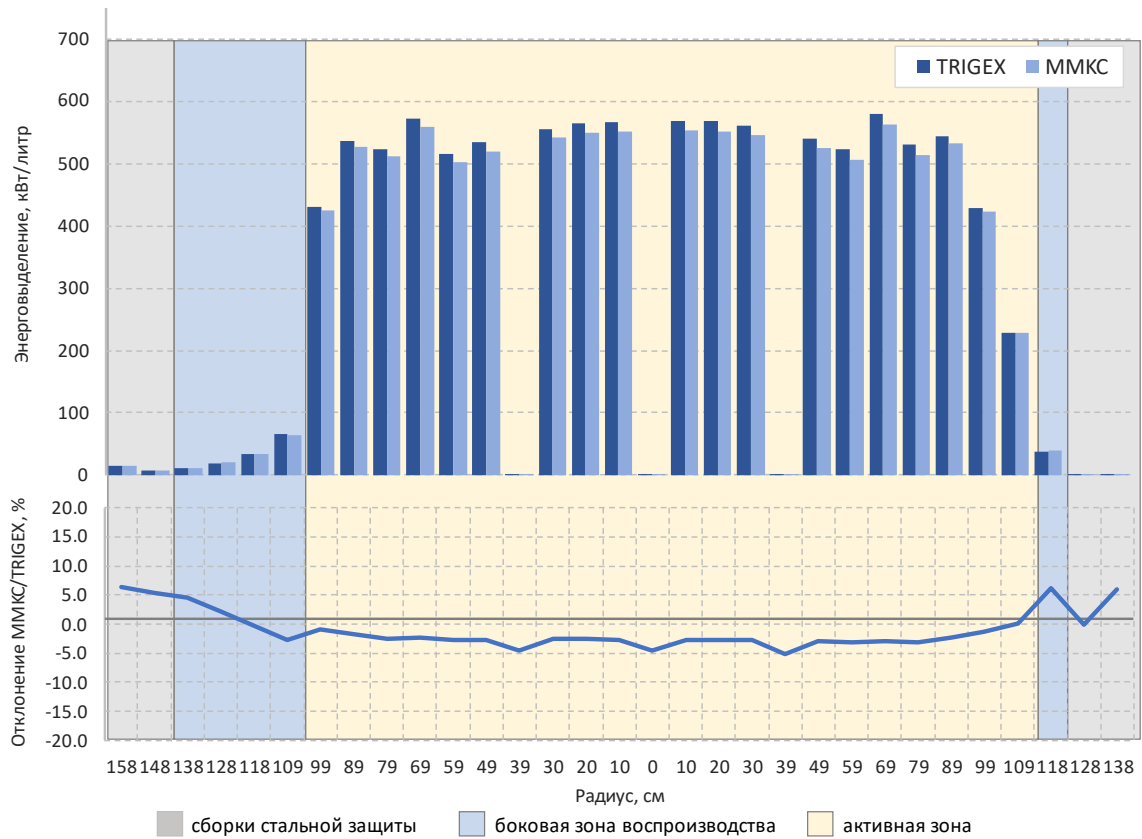
Рисунок 4.12 – Результаты методической поправки для удельного энерговыделения по радиусу активной зоны, 76 микрокампания РУ БН-600
