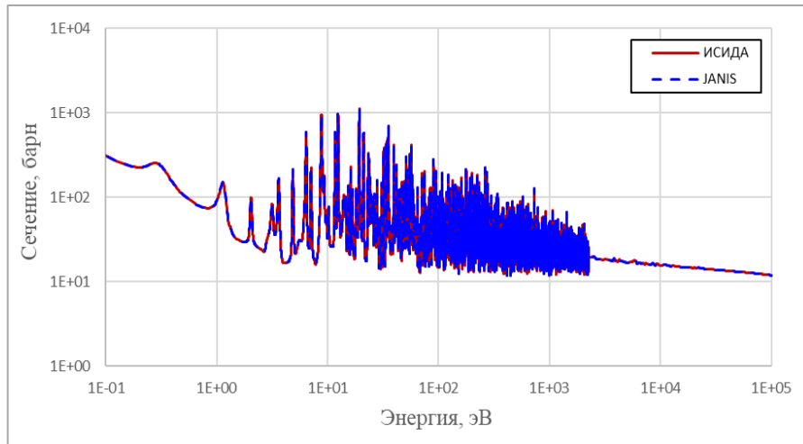
Рисунок 1.7 – Сравнение справочных данных ИСИДА и JANIS
