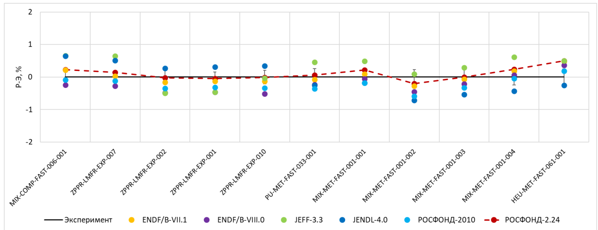
Рисунок 3.8 – Расчетно-экспериментальное отклонение k_{эф} для сборок ZPPR (топливо – Pu, МОКС)
