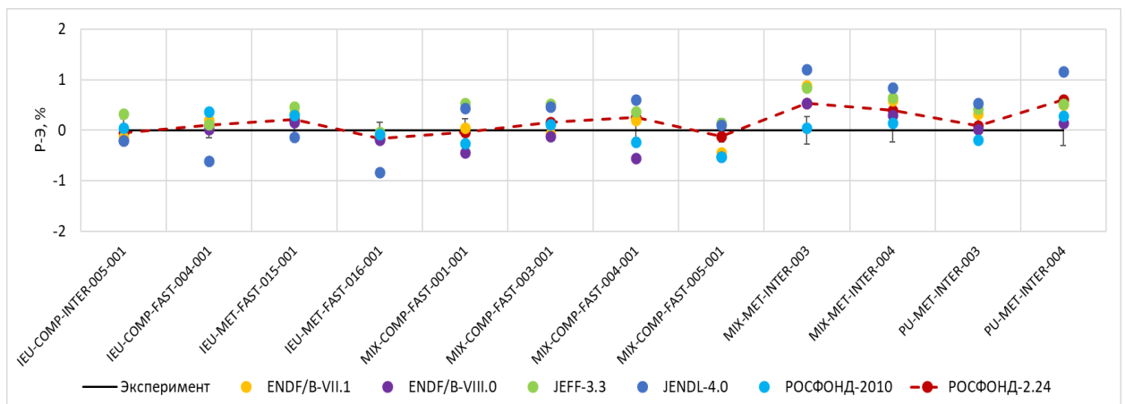
Рисунок 3.7 – Расчетно-экспериментальное отклонение k_{эф} для сборок ZPR (топливо – UO_2 , МОКС)
