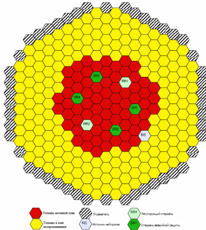
Рисунок 2.16 – Картограмма активной зоны реактора JOYO
