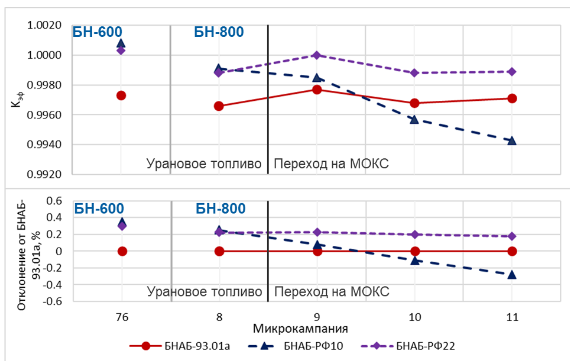
Рисунок 4.3 – Результаты расчета k_{эф} реакторов БН-600, БН-800 и отклонение от БНАБ-93.01а
