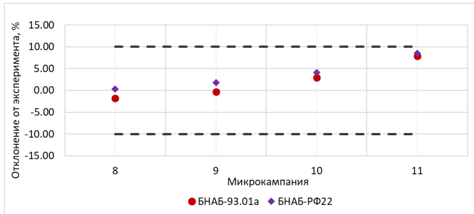
Рисунок 4.5 – Средние значения расчетно-экспериментальных отклонений эффективности стержней АЗ
