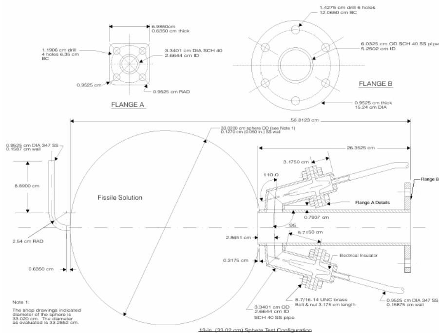
Рисунок 2.5 – Схема поперечного среза конфигурации PU-SOL-THERM [38]
