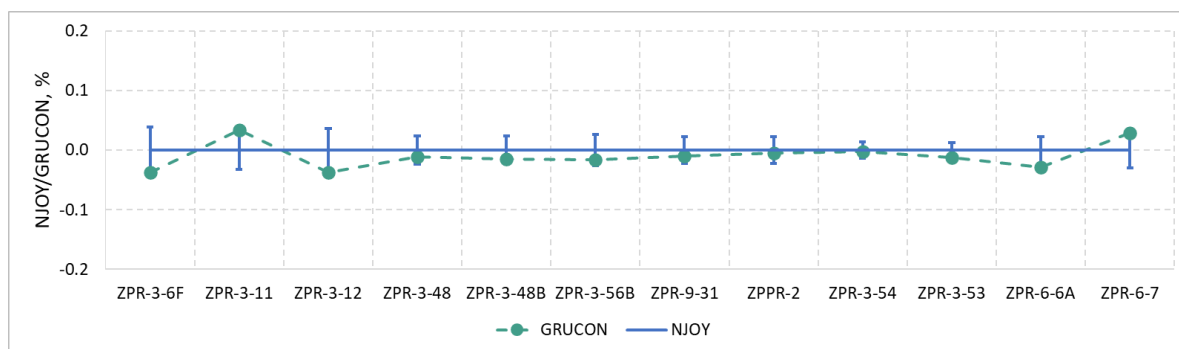
Рисунок 3.4 – Расхождение значений критичности для РС
