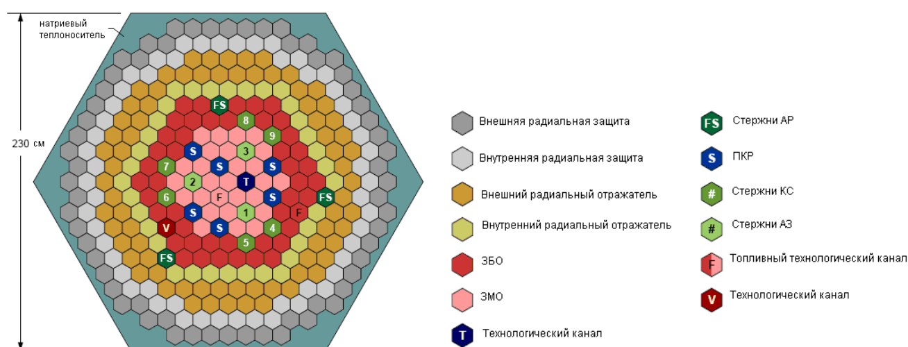
Рисунок 2.15 – Компоновка активной зоны реактора FFTF
