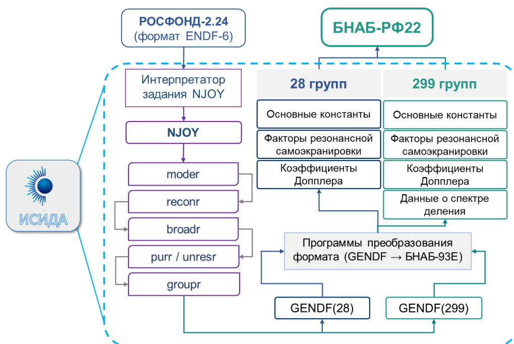
Рисунок 4.2 – Схема процесса подготовки групповых констант
