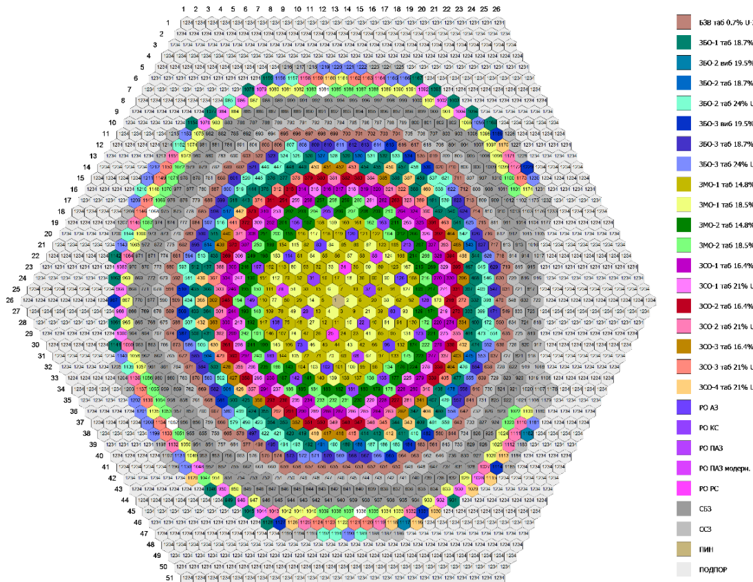
Рисунок 2.13 – Картограмма реактора БН-800 (10 микрокампания)
