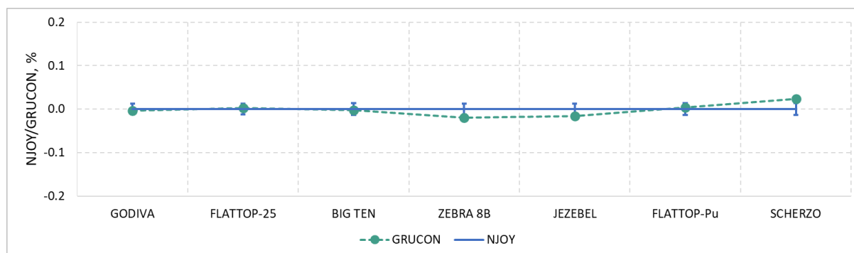
Рисунок 3.3 – Расхождение значений критичности для КМС
