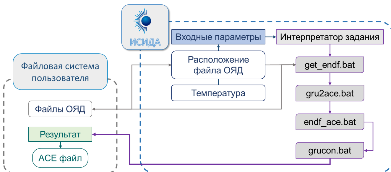
Рисунок 3.2 – Схема подготовки ACE файлов с помощью GRUCON
