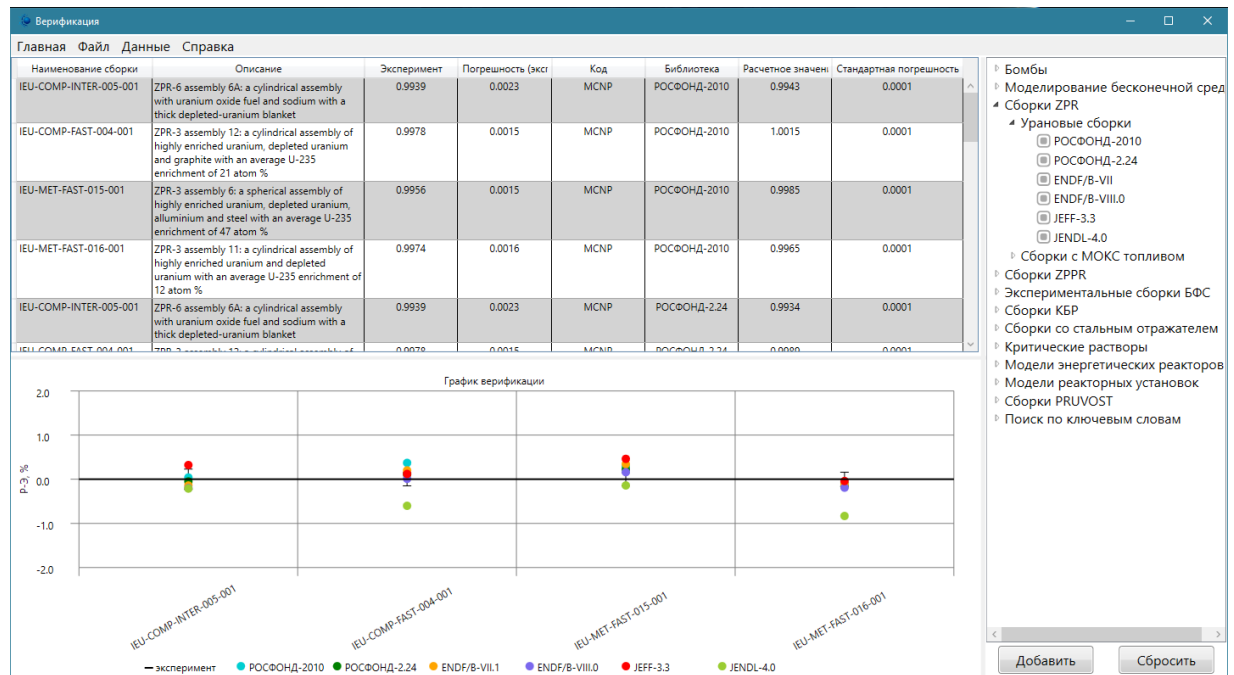
Рисунок 1.10 – Интерфейс рабочей среды «Верификация»
