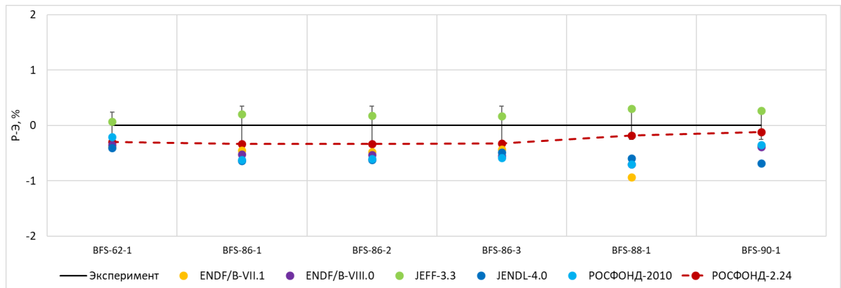
Рисунок 3.10 – Расчетно-экспериментальное отклонение k_{эф} для сборок БФС с натриевым теплоносителем
