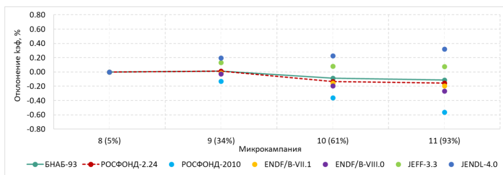
Рисунок 3.12 – Изменение значения k_{эф} по отношению к 8 микрокампании реактора БН-800
