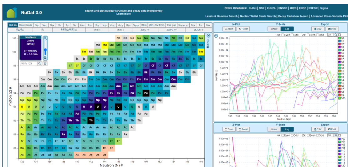
Рисунок 1.12 – Веб-интерфейс NNDC [43]
