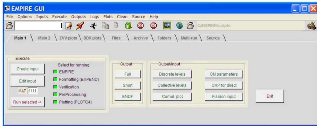
Рисунок 1.16 – Интерфейс EMPIRE [27]
