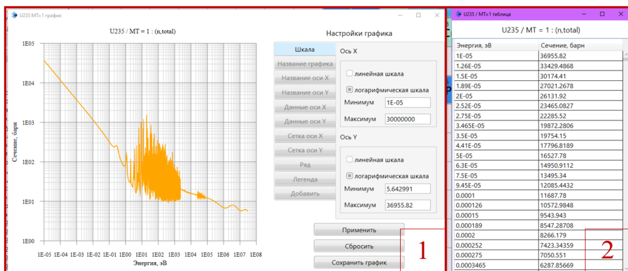
Рисунок 1.4 – Представление зависимости полного сечения от энергии для U-235
