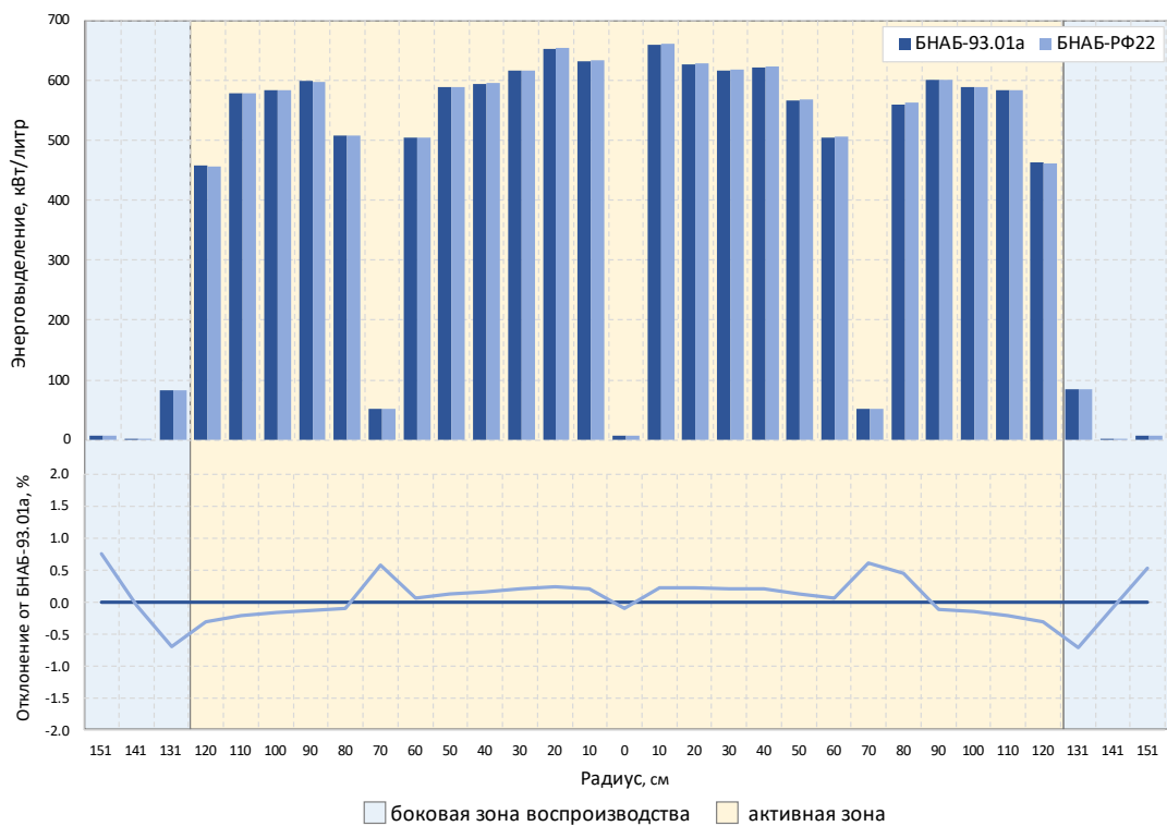
Рисунок 4.11 – Результаты расчета удельного энерговыделения по а.з. реактора БН-800 по системам констант БНАБ-93.01а и БНАБ-РФ22
