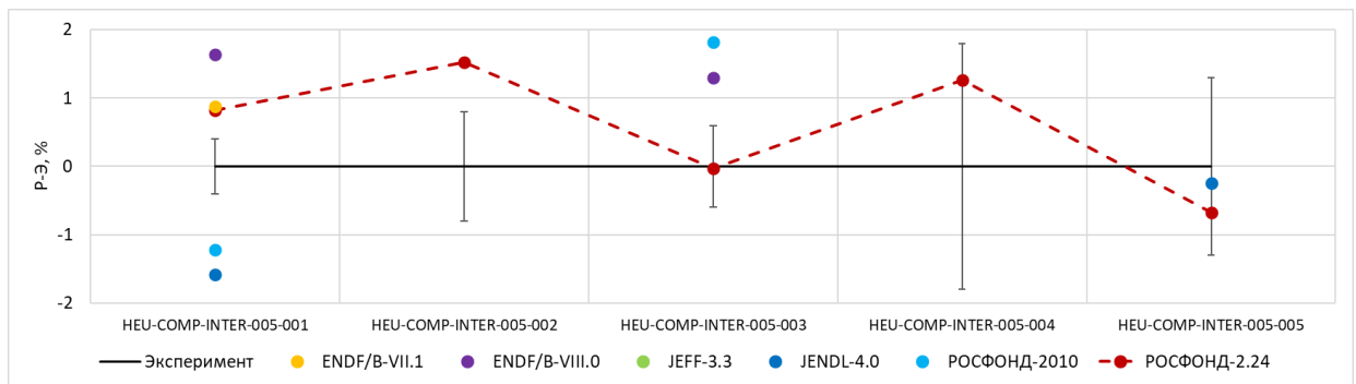
Рисунок 3.9 – Расчетно-экспериментальное отклонение k_{эф} для сборок KBR
