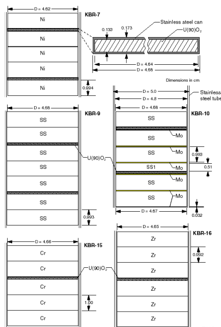
Рисунок 2.4 – Составы ячейки исследуемой зоны для критических сборок KBR-7, -9, -10, -15, и -16 [37]
