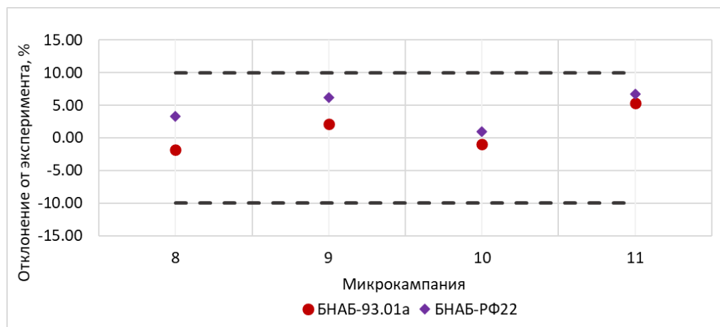
Рисунок 4.8 – Средние значения расчетно-экспериментальных отклонений эффективности стержней РС
