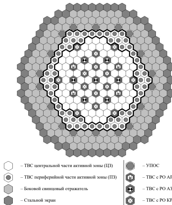
Рисунок 2.18 – Картограмма активной зоны реактора БРЕСТ-ОД-300
