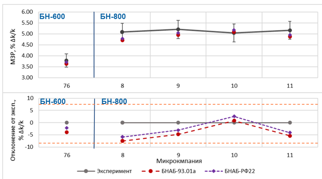
Рисунок 4.4 – Результаты расчета запаса реактивности реакторов БН-600, БН-800
