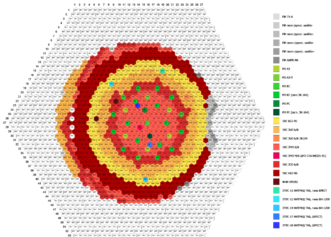
Рисунок 2.8 – Картограмма реактора БН-600 (77 микрокампания)
