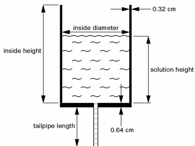
Рисунок 2.6 – Экспериментальная конфигурация NEU-SOL-TERM [38]
