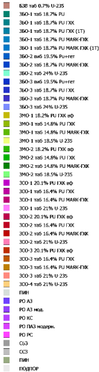
Рисунок 2.14 – Картограмма реактора БН-800 (11 микроампания)
