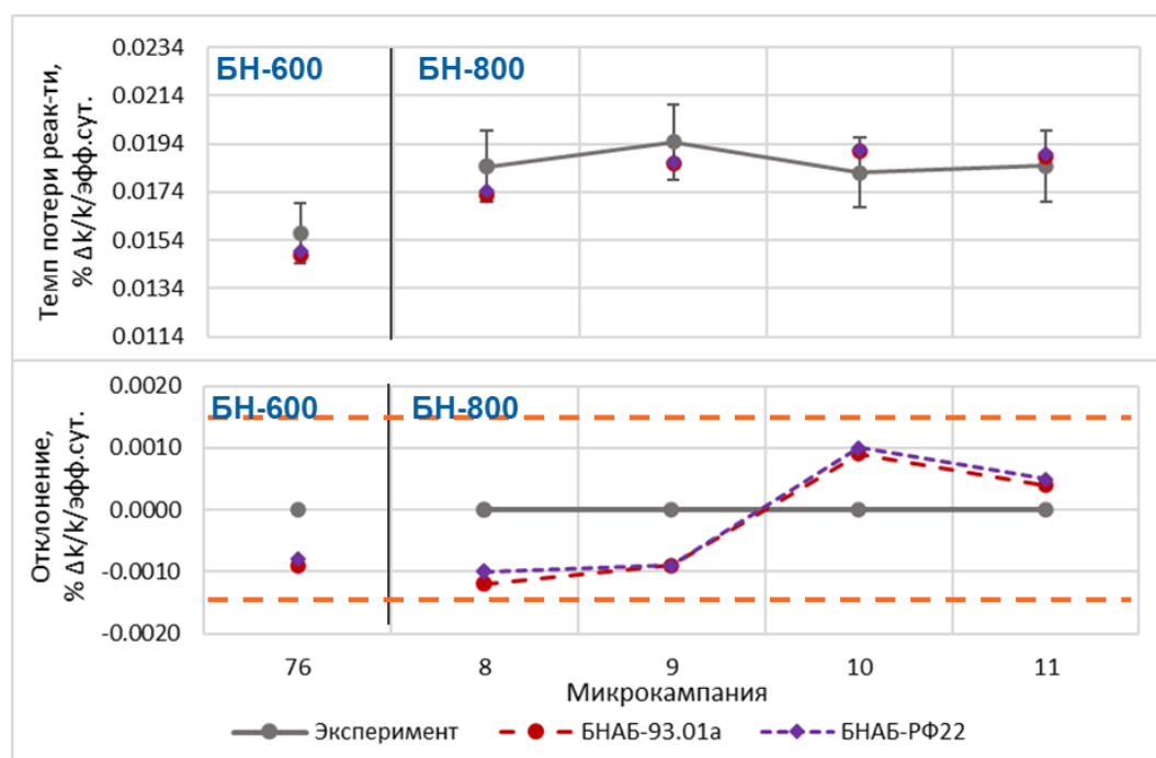
Рисунок 4.9 – Результаты расчета и расчетно-экспериментальные отклонения темпа потери реактивности за микроампанию
