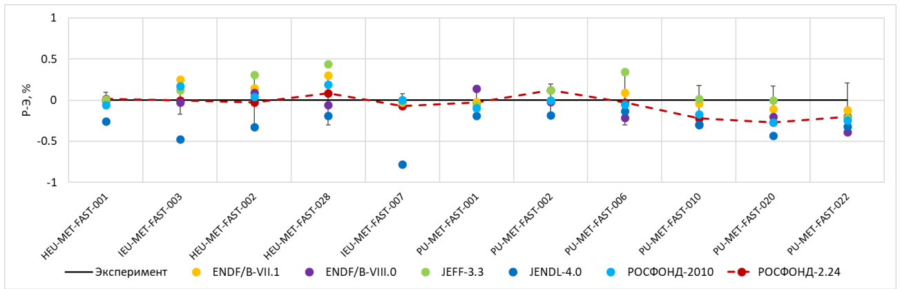
Рисунок 3.5 – Расчетно-экспериментальное отклонение k_{эф} (бомбы)
