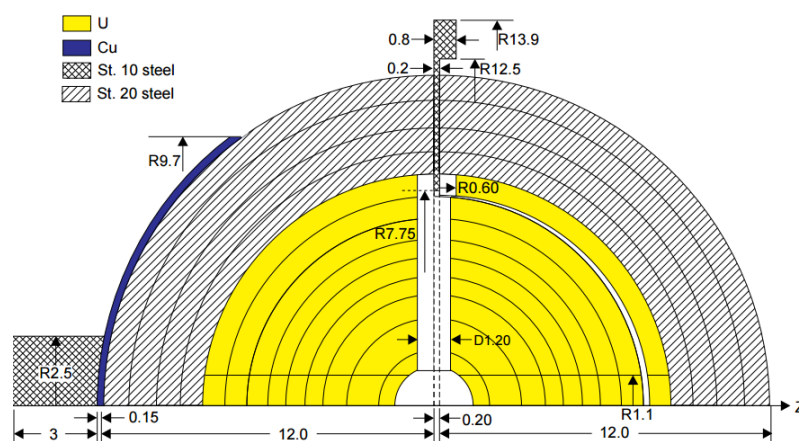
Рисунок 2.2 – Сферическая конфигурация (HEU-MET-FAST-013) [37]
