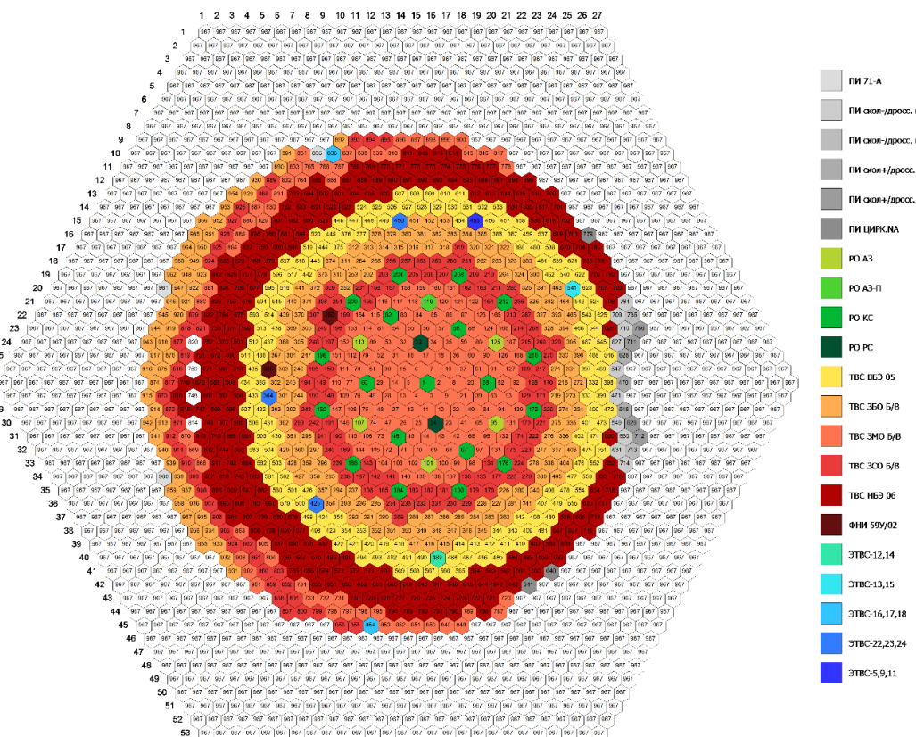
Рисунок 2.10 – Карттограмма реактора БН-600 (79 микроампания)
