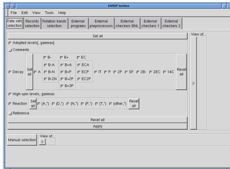
Рисунок 1.15 – Интерфейс ENSDF_toolbox [26]
