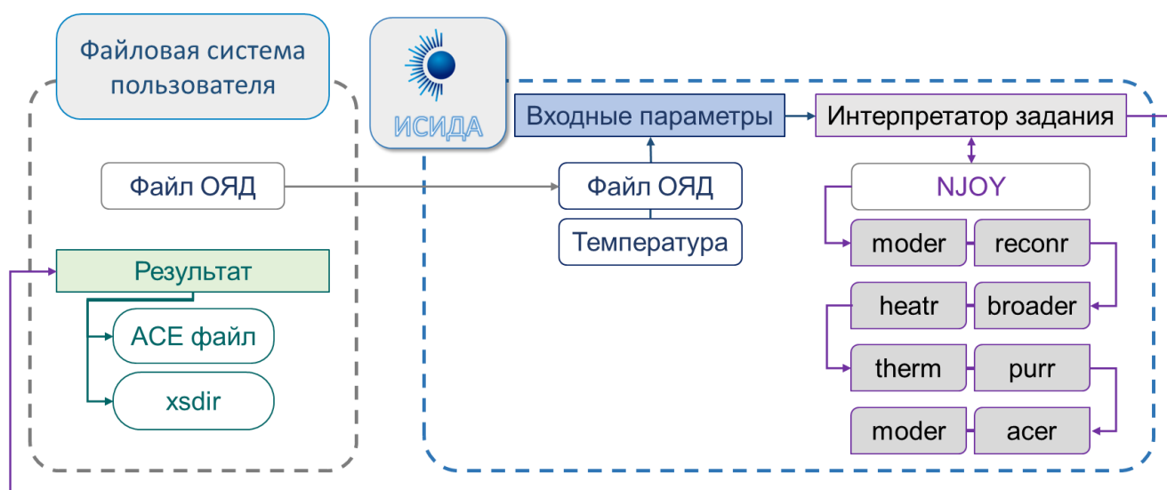
Рисунок 3.1 – Схема подготовки ACE файлов с помощью NJOY
